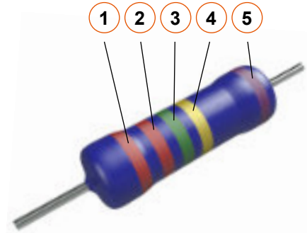
Beispiel: 22,50hm, ±0,1%
